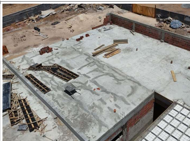
Foto 5 – Execução de laje treliçada (superestrutura)
