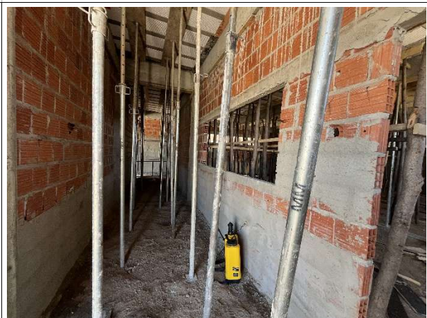
Foto 14 – Impermeabilização de alvenaria
