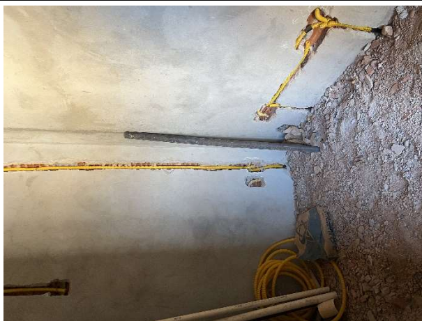
Fig. 11 – Execução de instalações elétricas da guarita
