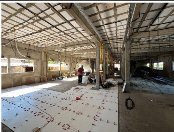
Fig. 5 – Execução de piso e instalações
