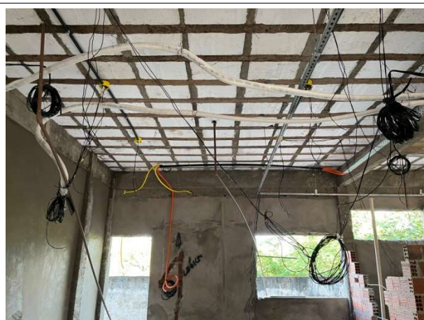
Fig. 12 – Laje treliçada (superestrutura) e instalações
