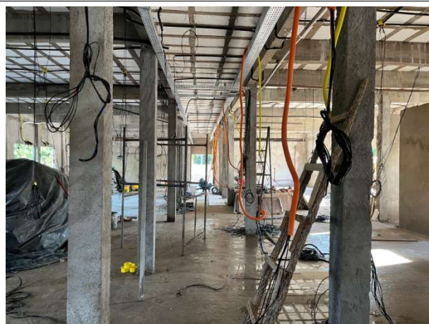
Fig. 10 – Execução de instalações elétricas e lógicas
