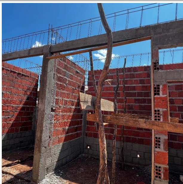
Fig. 7 – Execução de pilares e vigas.
