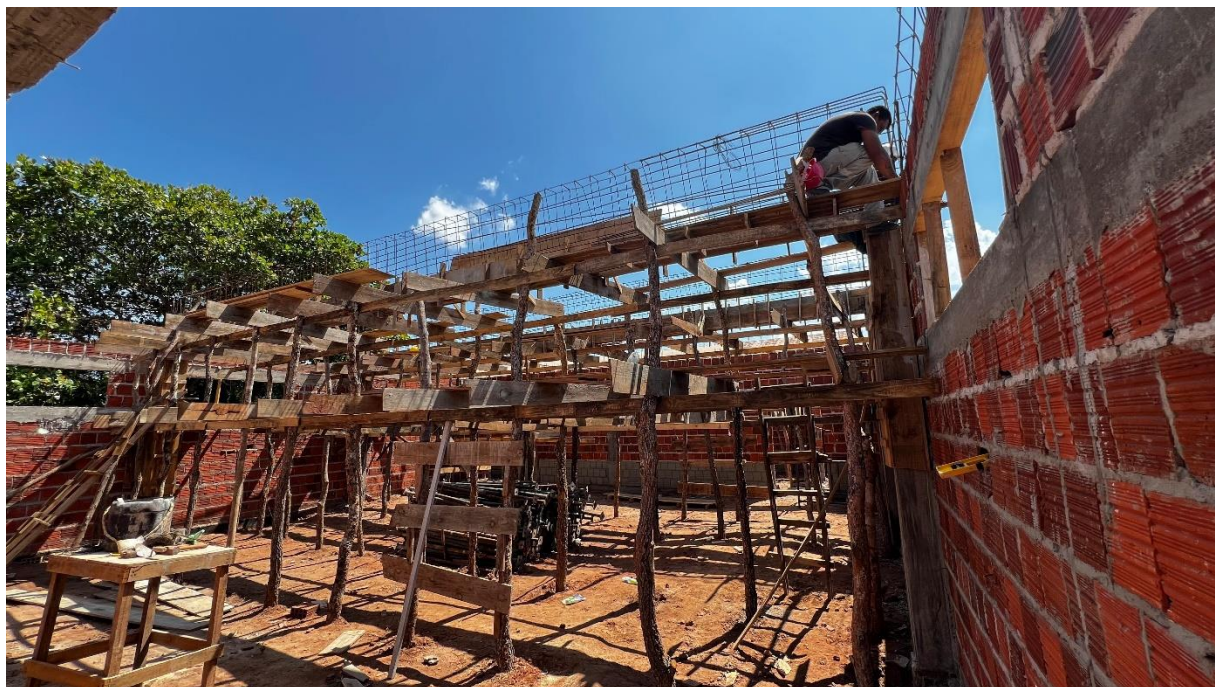
Fig. 10 – Armação para vigas.
