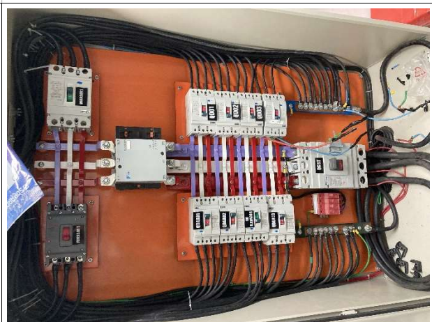
Fig. 14 – Quadro geral de baixa tensão
