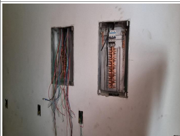
Fig. 13 – Instalações Elétricas/Lógicas
