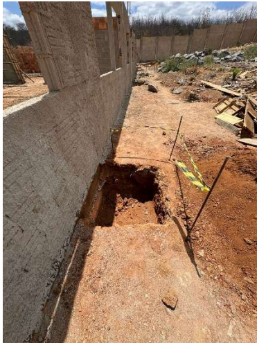
Fig. 11 – (10.0 Instalações Hidrossanitárias)
