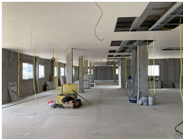
Fig. 9 – execução de forro, instalações elétricas e lógicas
