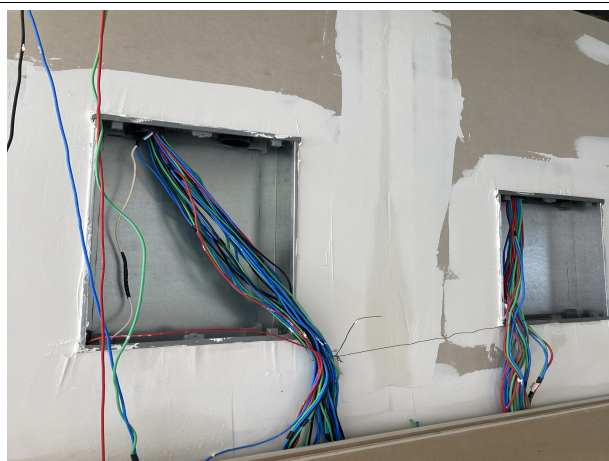
Fig. 13 – execução de instalações elétricas
