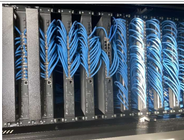
Fig. 12 – instalações de cabeamento estruturado
