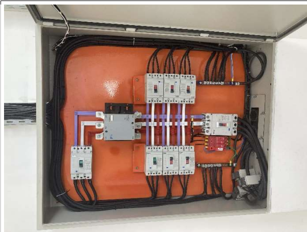
Fig. 15 – quadro geral de baixa tensão
