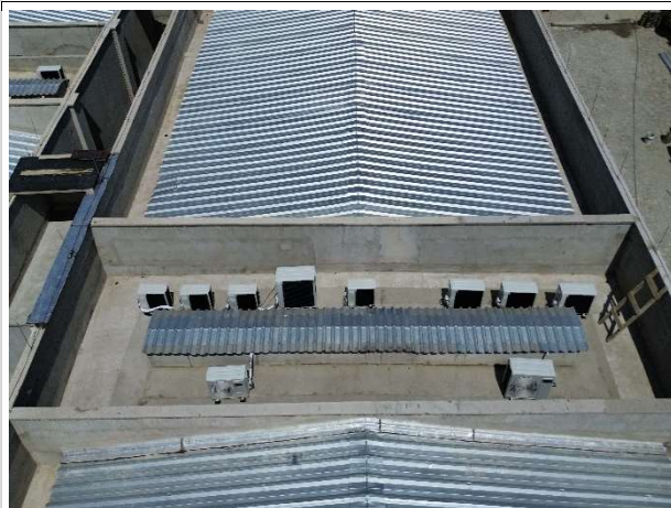
Fig. 17 – condensadoras (ar condicionado)
