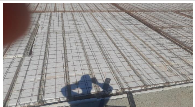
Fig. 16 – Superestrutura/Lajes
