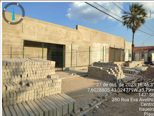
Fig. 11 – execução de pavimento intertravado
