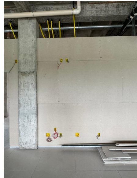
Foto 4 – Divisória de gesso acartonado e instalações elétricas e de lógica EJUD
