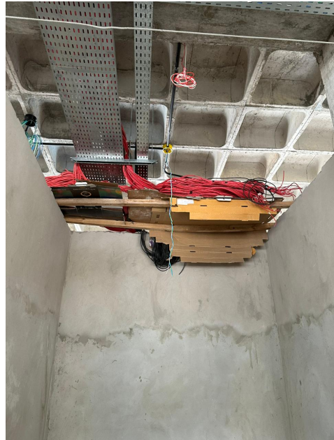
Foto 18 – Instalações de lógica Corregedoria
