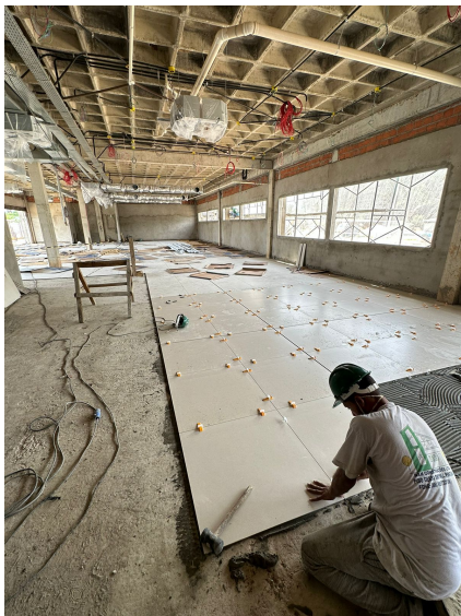
Foto 11 – Revestimento cerâmico Corregedoria
