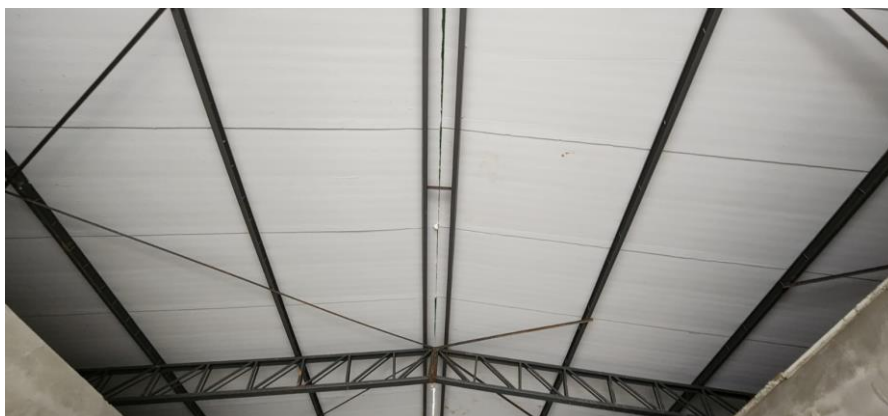
FOTO 2 – COBERTURA - INSTALAÇÃO DE TESOURA, ESTRUTURA METÁLICA, TRAMA DE AÇO COMPOSTO, TELHAMENTO
