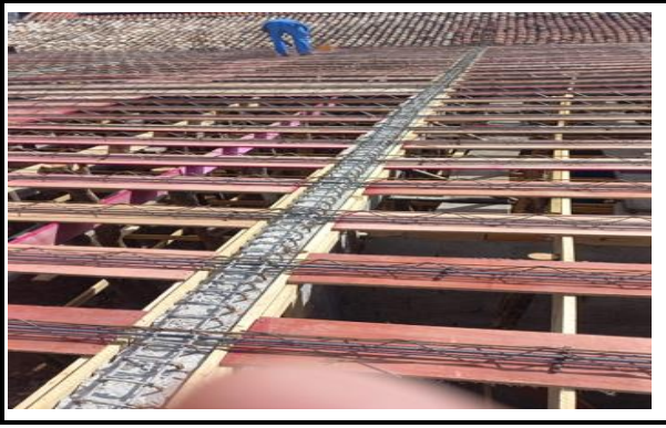
MONTAGEM FORMA/ARMADURA (LAJE)
